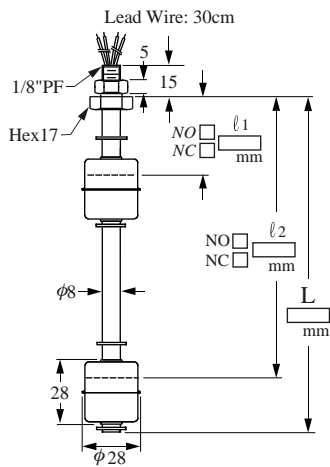
Washer: NBR
